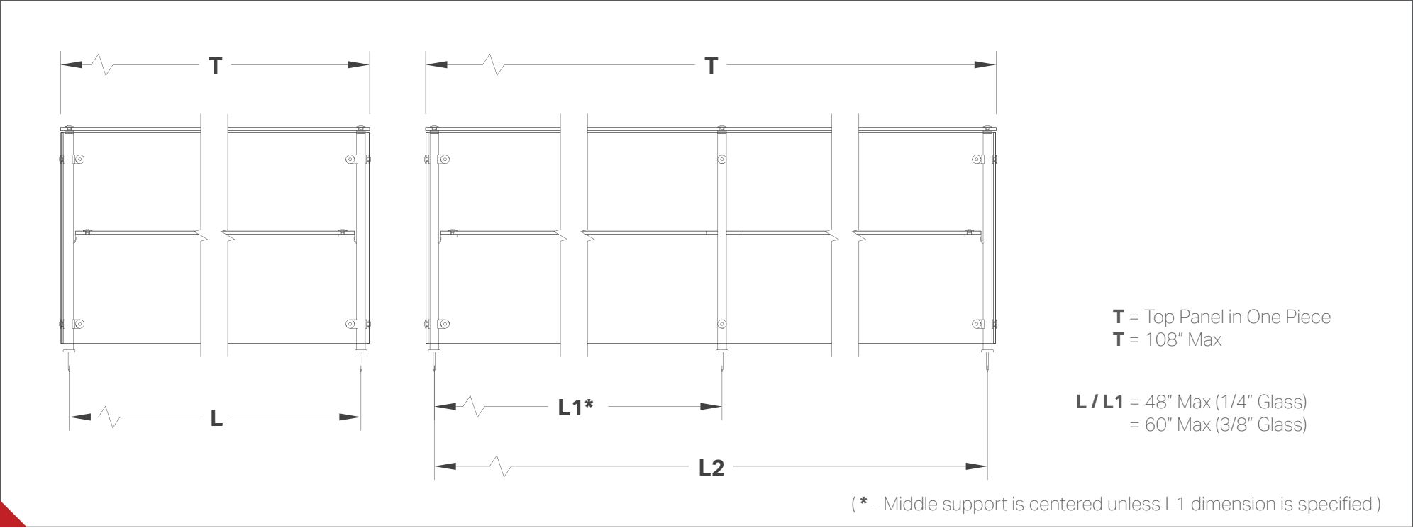
/////////////////CENTERLINE DIMENSIONS
